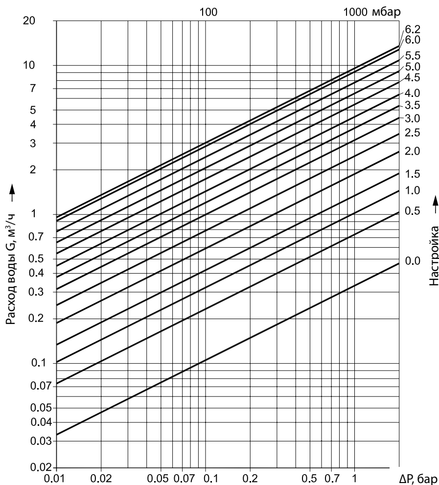
Диаграмма для настройки клапана Leno™ MSV-BD D_v = 25 мм
