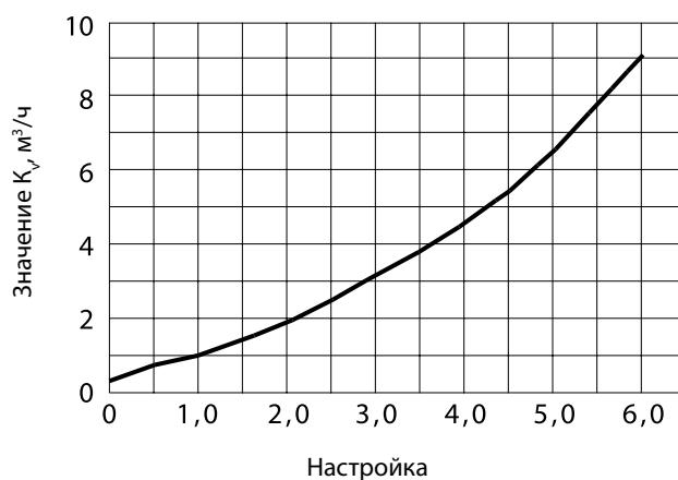
Расходная характеристика
